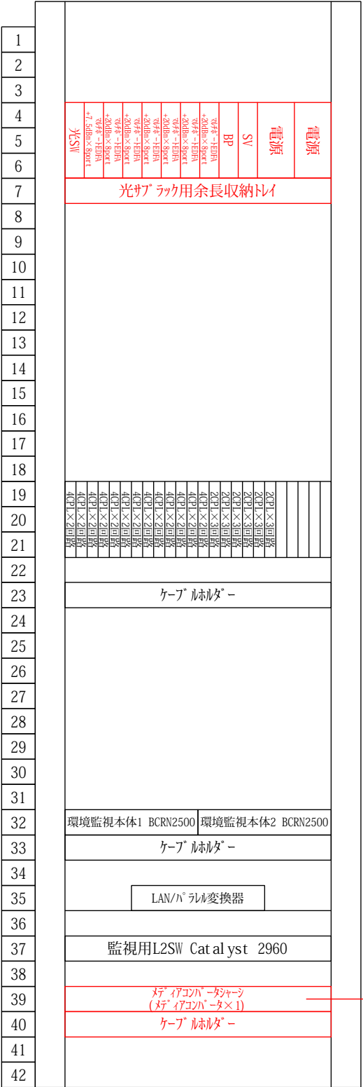
放送架 No. 1 (W700×H2000×D800)
